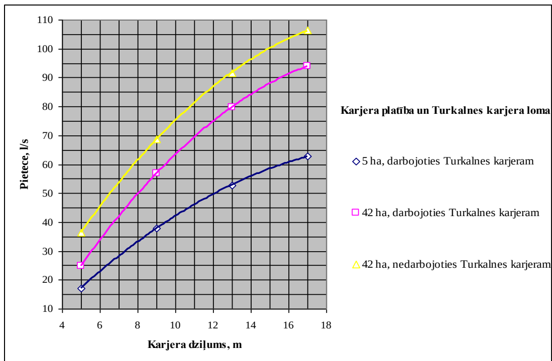
3.10. attēls. Pazemes ūdeņu pietece karjerā atkarībā no tā dziļuma, platības un ūdens atsūkņēšanas režīma Tūrkalnes karjerā
