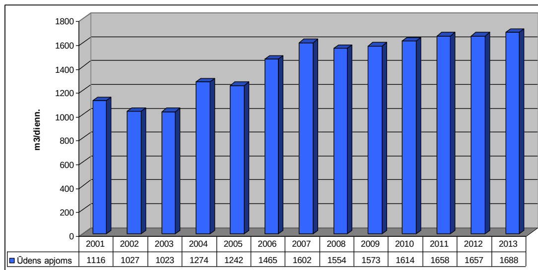
3.13.att. Vidējais atsūkņētais ūdens apjoms diennaktī (2001 - 2013)
