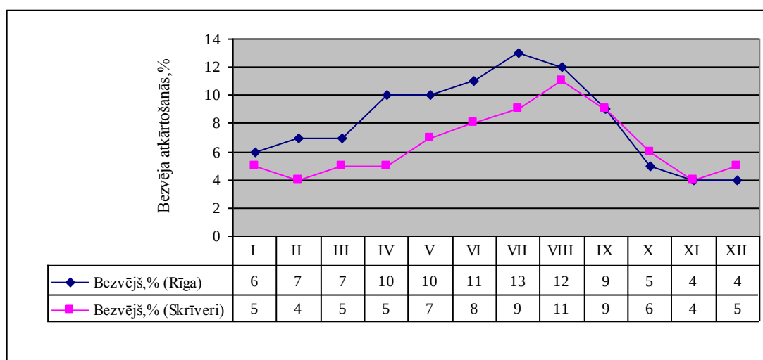
2.11.attēls. Bezvēja atkārtošanās, %
