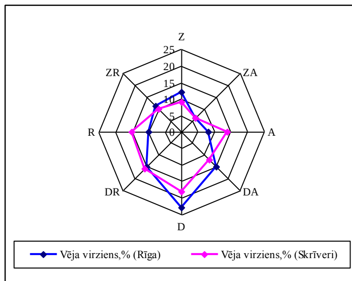
2.9.attēls. Vēja virzienu atkārtošanās gadā, %
